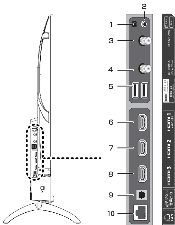
側面 入出力端子部
